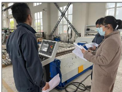
图二 卷板机性能安全检查
